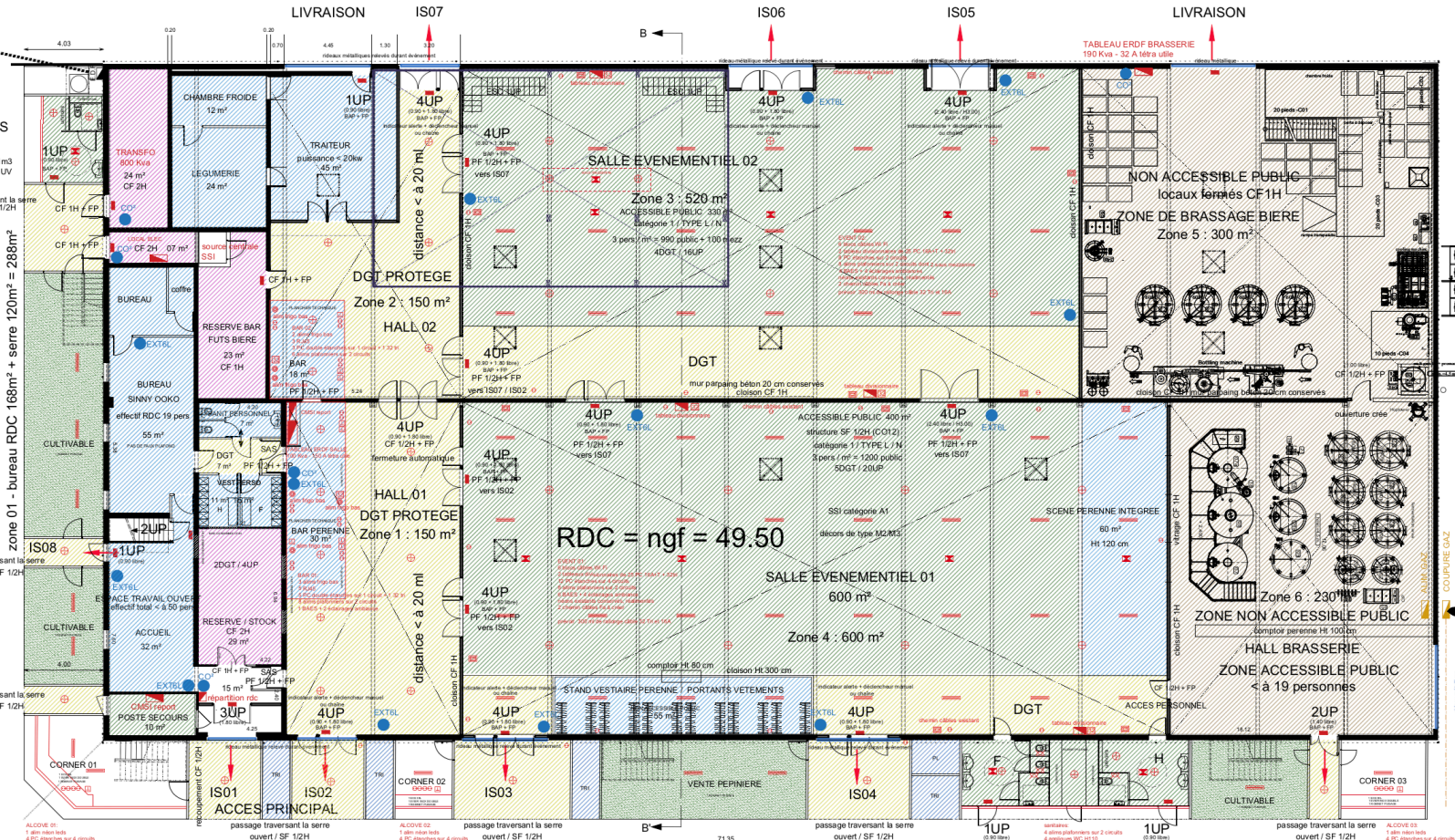
PLAN RDC - BÂTIMENT DIVA
